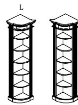
УГЛОВОЙ КОРПУС ШКАФА [PV 435222L] Ш: 43,5 / Г: 43,5 / В: 222 [PV 435222R] Ш: 43,5 / Г: 43,5 / В: 222
