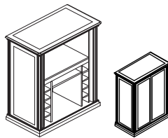
ШКАФ-БАР СО СКЛАДНЫМИ ДВЕРКАМИ [PV BAR] Ш: 110 / Г: 60 / В: 141
