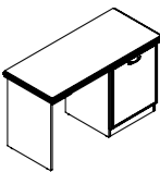
СТОЛ С ПРАВОЙ ТУМБОЙ ПОД ФРИГОБАР (GRN410DX) Ш: 1275 / Г: 560 / В: 750
