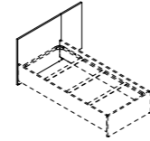
ИЗГОЛОВЬЕ КРОВАТИ ОДНОСПАЛЬНОЙ (VG220) Ш: 981 / Г: 18 / В: 910
