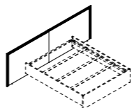
ИЗГОЛОВЬЕ КРОВАТИ ДВУСПАЛЬНОЙ И ТУМБ (GRN240) Ш: 2860 / Г: 35 / В: 1007
