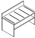
ТУМБА БАГАЖНАЯ (VG340) Ш: 900 / Г: 520 / В: 587
