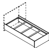
КАРКАС КРОВАТИ ОДНОСПАЛЬНОЙ С РЕШЕТКОЙ (VG110) Ш: 2045 / Г: 974 / В: 415
