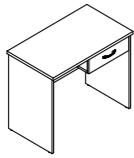
СТОЛ ТУАЛЕТНЫЙ С ПРАВЫМ ЯЩИКОМ (VG420DX) Ш: 900 / Г: 520 / В: 750
