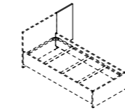
ПАНЕЛЬ ТУМБЫ (VG210) Ш: 470 / Г: 18 / В: 910
