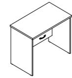
СТОЛ ТУАЛЕТНЫЙ С ЛЕВЫМ ЯЩИКОМ (VG420SX) Ш: 900 / Г: 520 / В: 750
