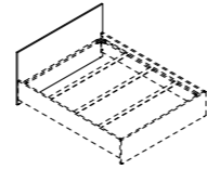
ИЗГОЛОВЬЕ КРОВАТИ ДВУСПАЛЬНОЙ И ТУМБ (VG230) Ш: 981 / Г: 18 / В: 910
