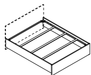
КАРКАС КРОВАТИ ДВУСПАЛЬНОЙ С РЕШЕТКОЙ (VG120) Ш: 2045 / Г: 1675 / В: 415
