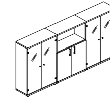
КОМПОЗИЦИЯ ШКАФОВ С НИШЕЙ (TAR904) Ш: 240 / Г: 36 / В: 117
