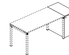
ОРГАУЭР НИЗКИЙ (TAR903) Ш: 39 / Г: 70 / В: 75
