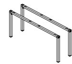
НАБОР КРАЙНИХ ОПОР ДЛЯ ДВОЙНОЙ СТОЛЕШНИЦЫ (TAR002) Ш: 144 / Г: 4 / В: 71
